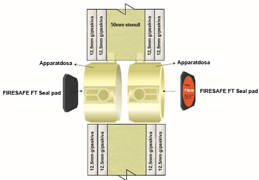
Väggdosor i gipsvägg monterade rygg mot rygg
