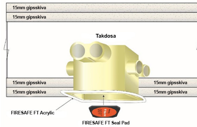
Takdosa monterad i gipstak
