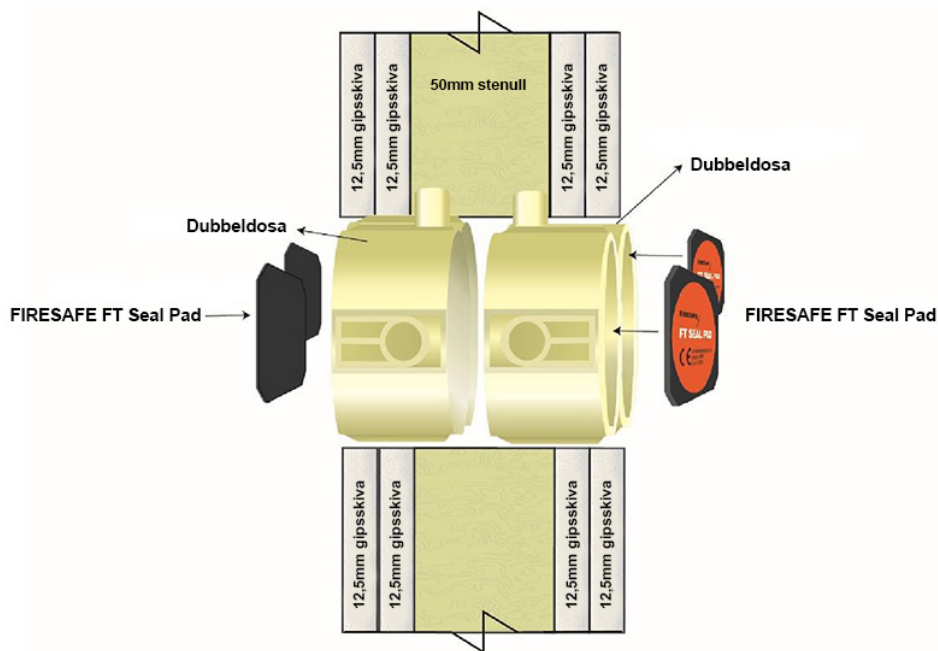
Dubbla väggdosor i gipsvägg monterade rygg mot rygg
