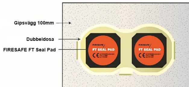
Dubbel väggdosa i gipsvägg, framifrån
