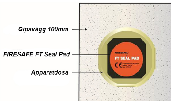
Väggdosa i gipsvägg, framifrån
