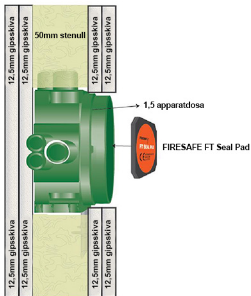
1,5 väggdosa monterad i gipsvägg
