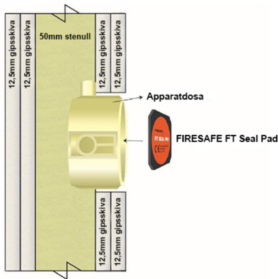
1-5st väggdosa monterade i rad på en sida av gipsvägg
