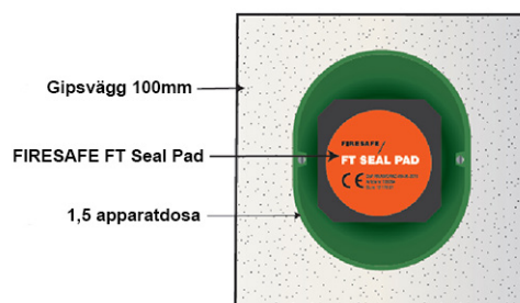
1,5 väggdosa monterade i gipsvägg, framifrån
