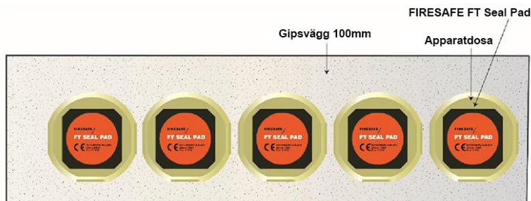
1-5st väggdosa monterade i rad på en sida av gipsvägg, framifrån
