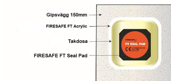
Takdosa monterad i gipstak, underifrån
